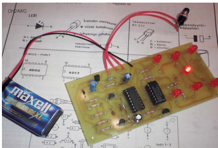
Elektroninen noppa.
