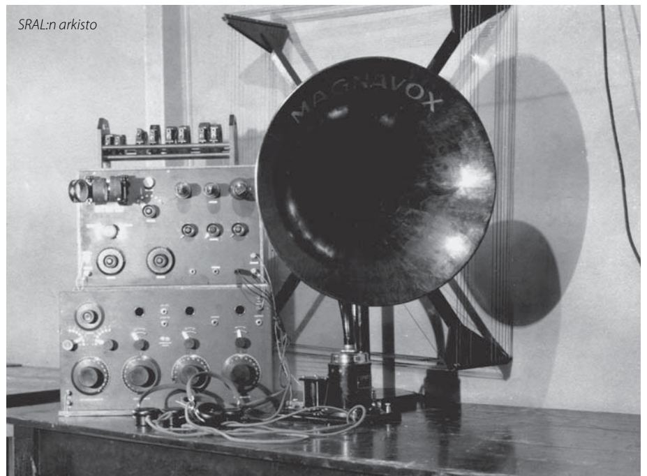
Radioamatööriasema 1930-luvulta.
